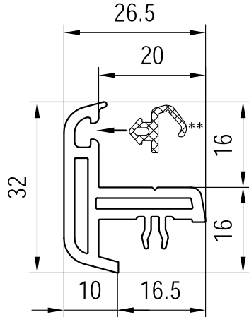
120x97 Schlagleiste -> SF-Mittel-Stoß (Schema C)
