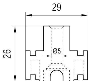
600098 Distanzstück, PVC, 100mm
